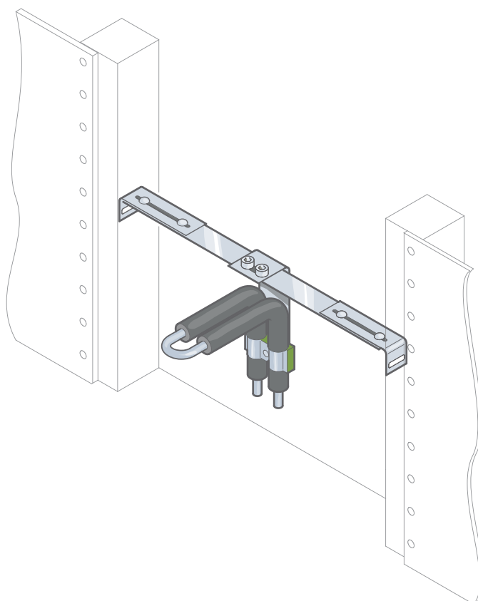
Montagesystem für Ventil-Kompaktheizkörper für verdeckten Wandanschluss: FIX KIT Trockenbau, montiert in Ständerwand
